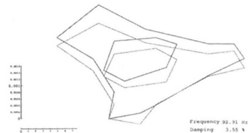
(d) Mode shape at 92.9 Hz
